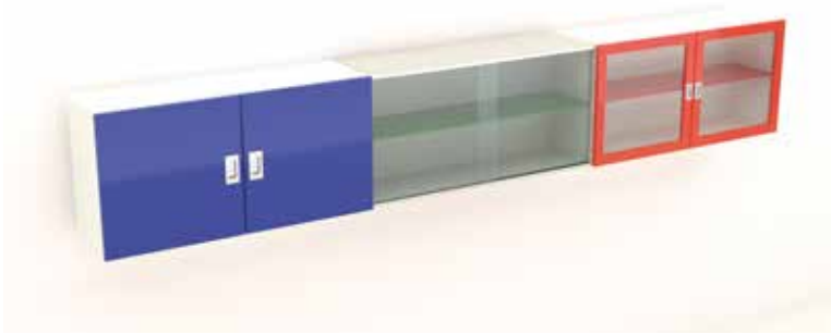
VITRINA DE COLGAR CON 2 PUERTAS CORREDIZAS Y/O ABATIBLES DE VIDRIO 6 mm SOBRE GUIAS DE ALUMINIO Y CARRETILLAS
